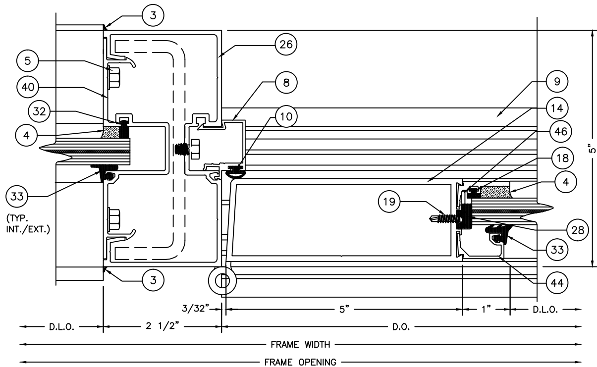
11 DOOR JAMB 10 SCALE: 6" = 1'-0"
