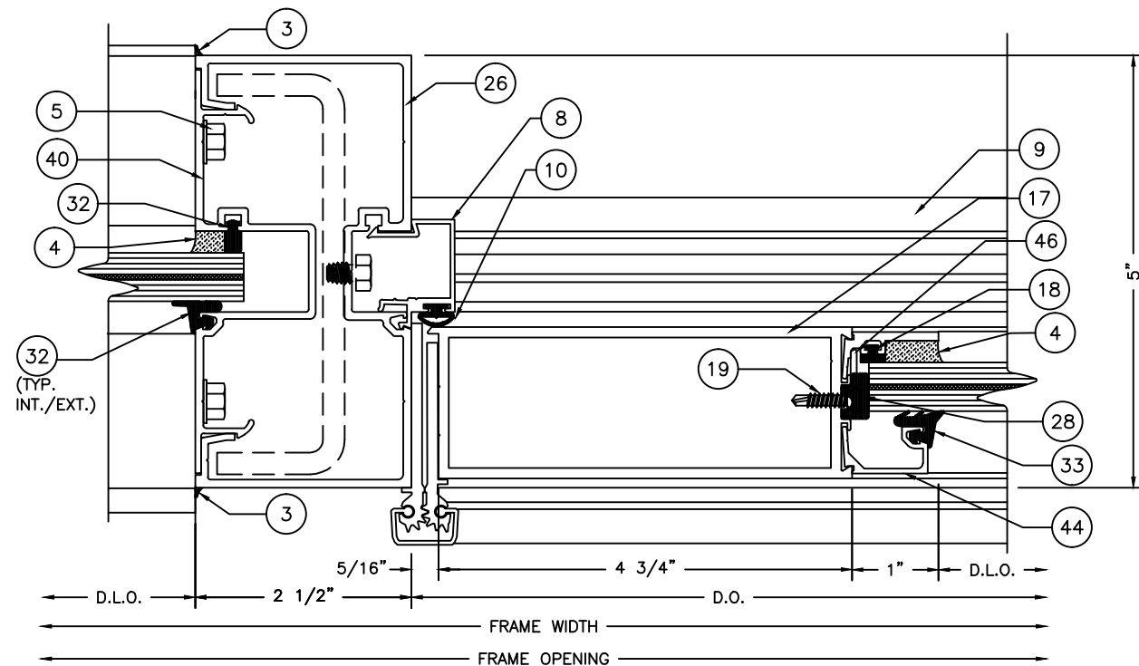
11 DOOR JAMB 10 SCALE: 6" = 1'-0"
