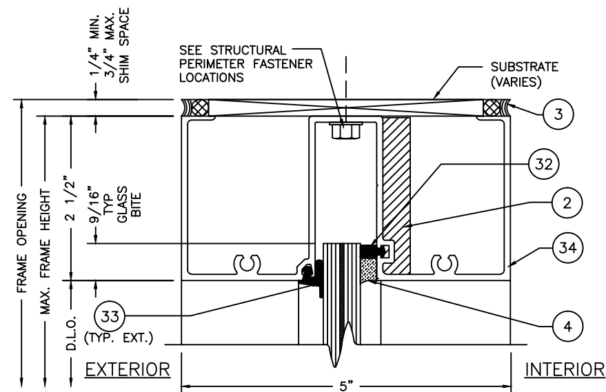
7 TRANSOM HEAD 9 SCALE: 6" = 1'-0"
