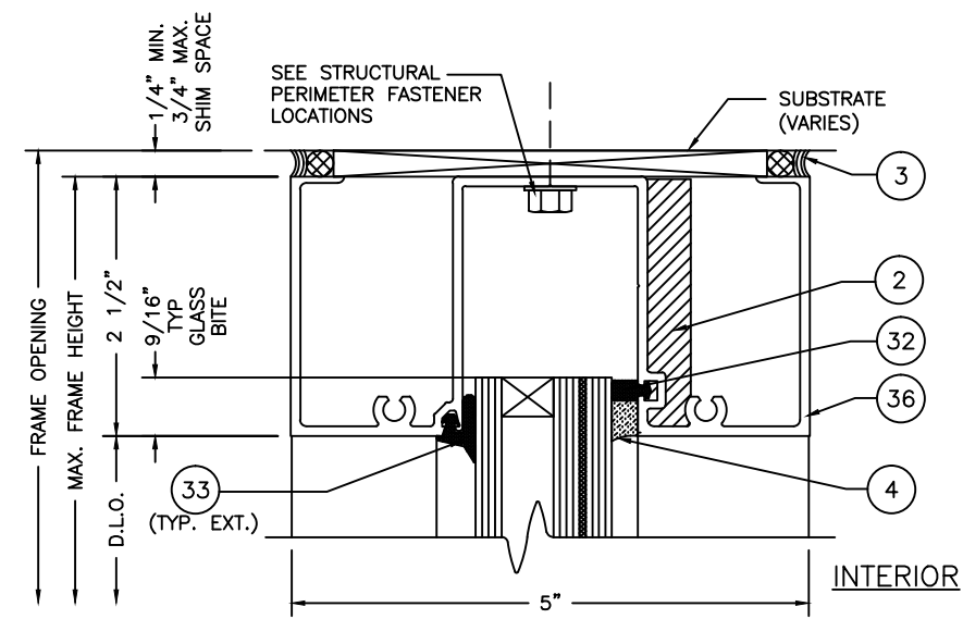
9 TRANSOM HEAD 9 SCALE: 6" = 1'-0"
