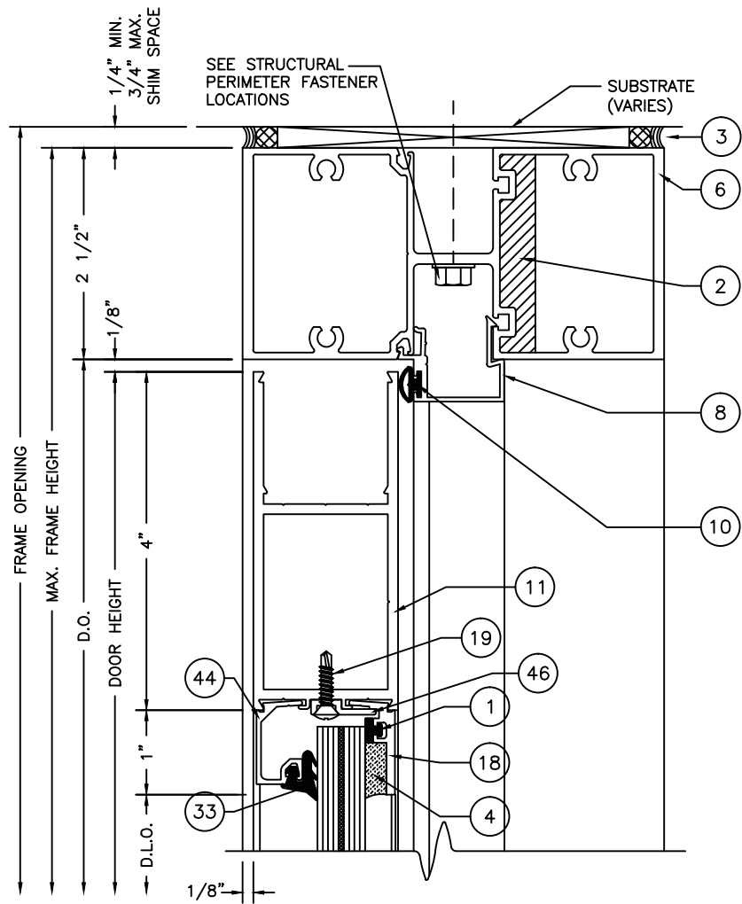
1 DOOR HEADER 7 SCALE: 6" = 1'-0"
