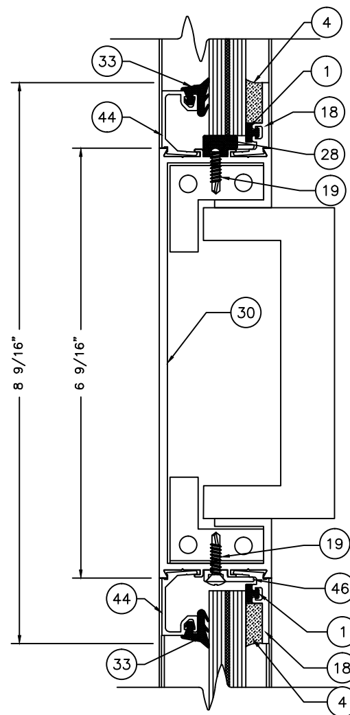
3 MID-PANEL PANIC 7 SCALE: 6" = 1'-0"
