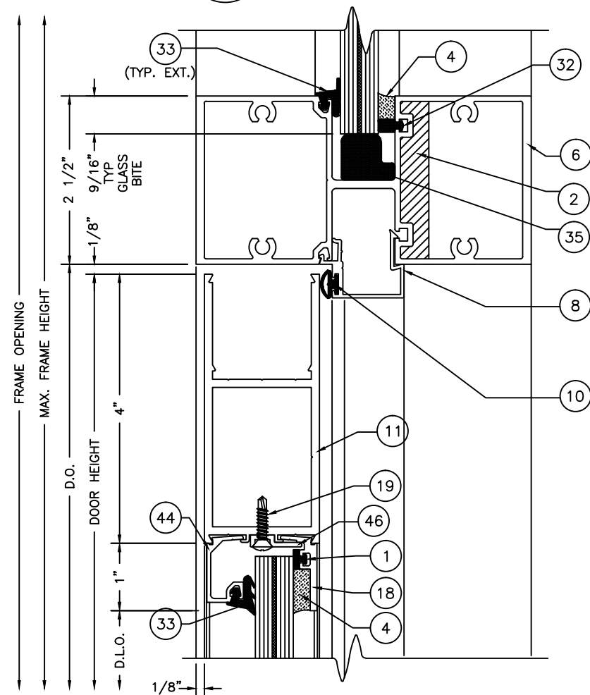
7 TRANSOM HEAD 9 SCALE: 6" = 1'-0"
