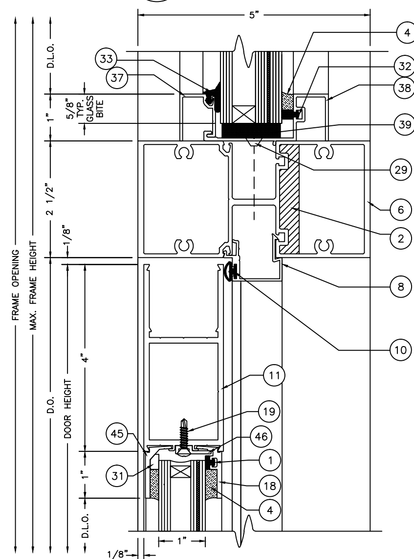
10 DOOR HEADER 9 SCALE: 6" = 1'-0"
