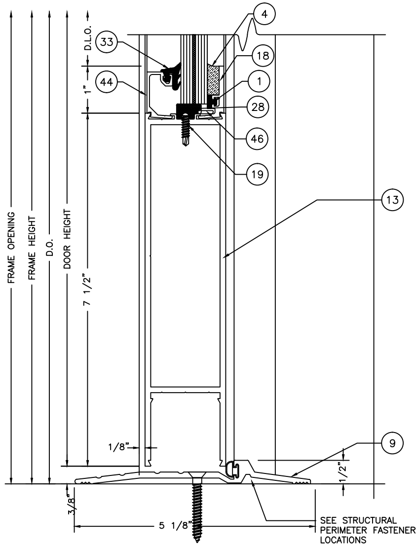
2 THRESHOLD 7 SCALE: 6" = 1'-0"
