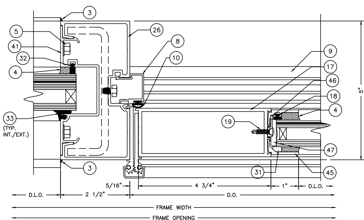
14 DOOR JAMB 10 SCALE: 6" = 1'-0"
