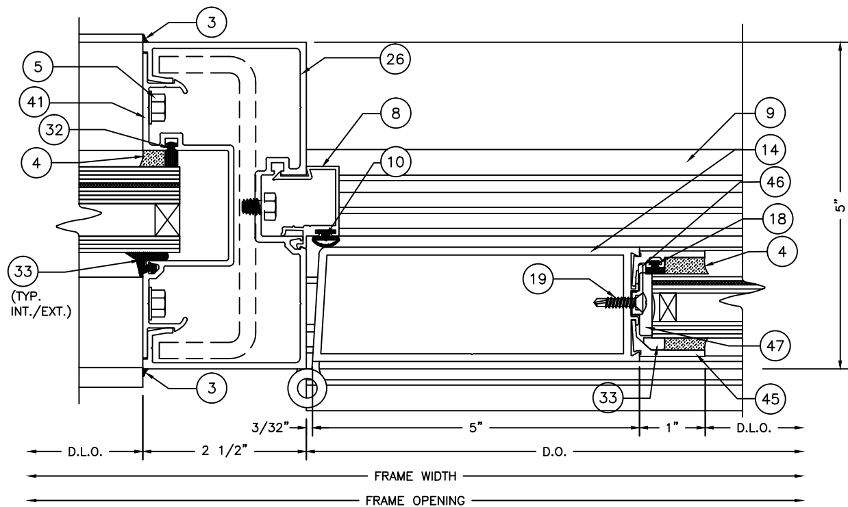
13 DOOR JAMB 10 SCALE: 6" = 1'-0"
